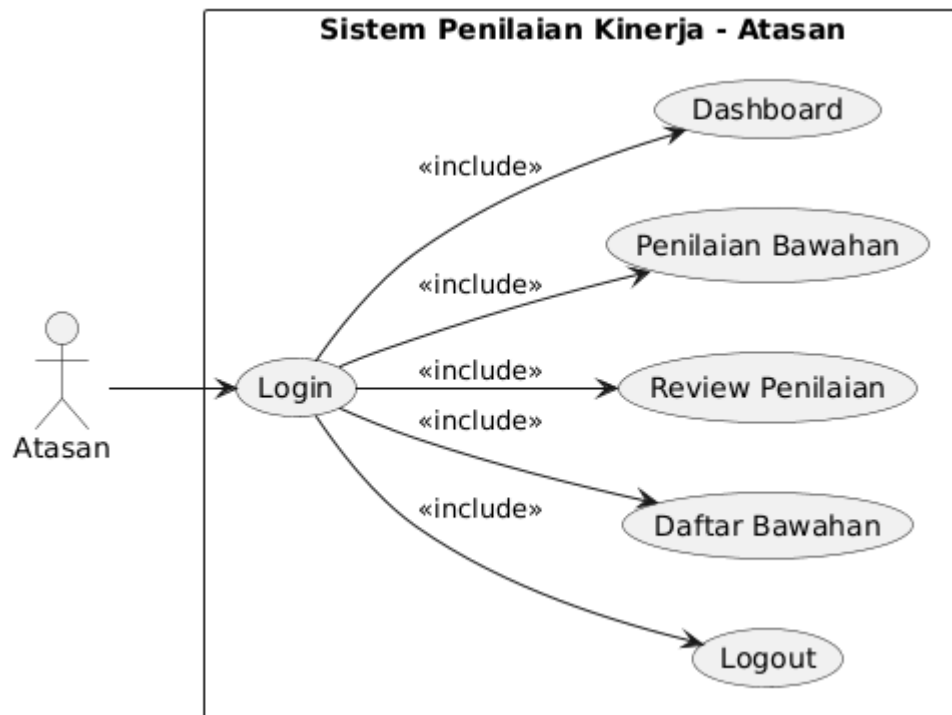
Gambar 4.2 Use case sistem untuk atasan Sumber : Hasil Rancangan
