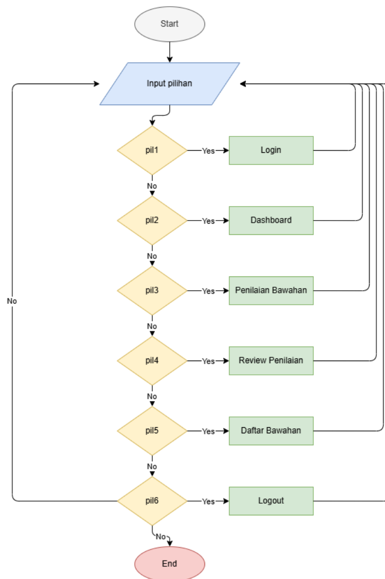
Gambar 4.48 flowchart Menu Atasan Sumber : Hasil Rancangan
