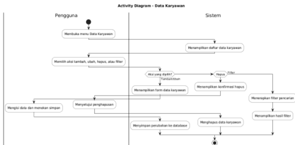
Gambar 4.8 Activity Diagram Data Karyawan Sumber : Hasil Rancangan
