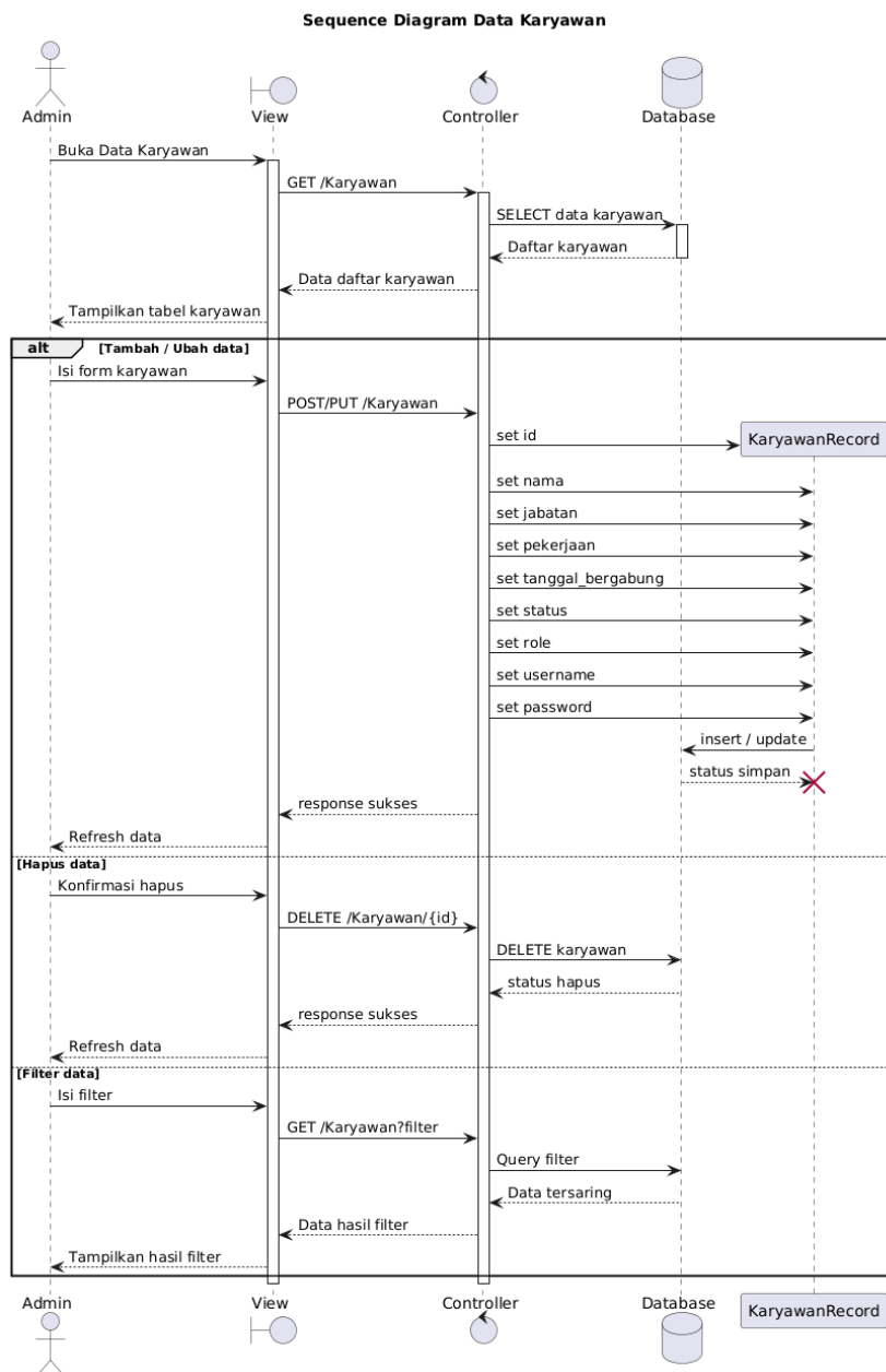
Gambar 4.23 Sequence Diagram Data Karyawan Sumber : Hasil Rancangan
