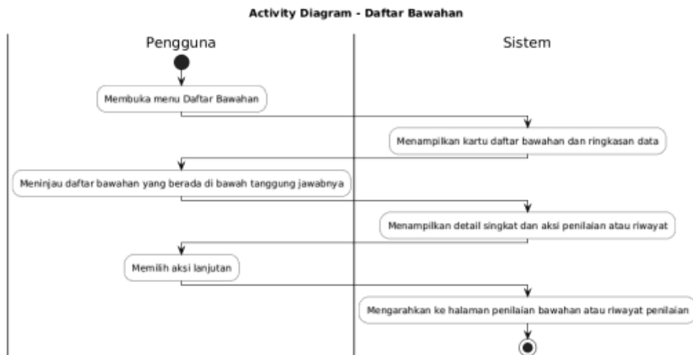
Gambar 4.16 Activity Diagram Daftar Bawahan Sumber : Hasil Rancangan
