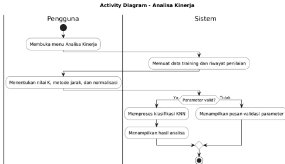
Gambar 4.13 Activity Diagram Analisa Kinerja Sumber : Hasil Rancangan
