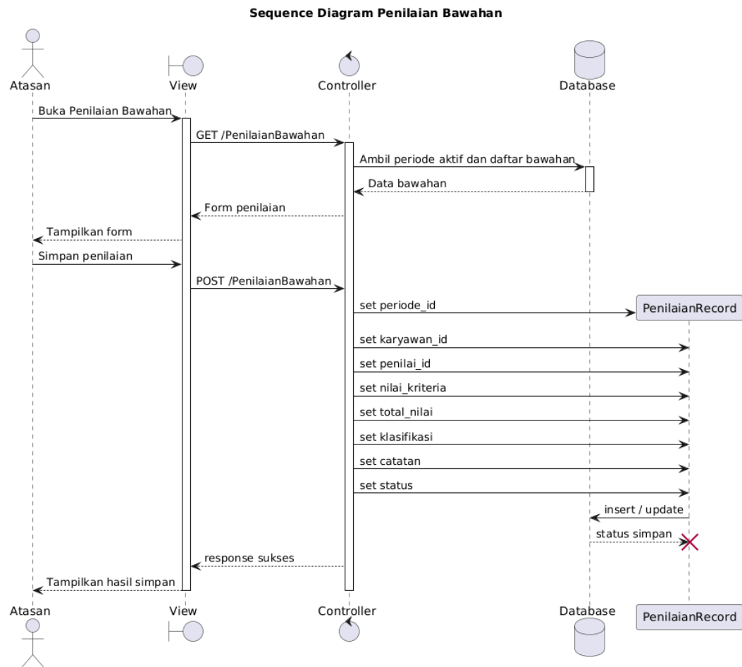
Gambar 4.29 Sequence Diagram Penilaian Bawahan Sumber : Hasil Rancangan
