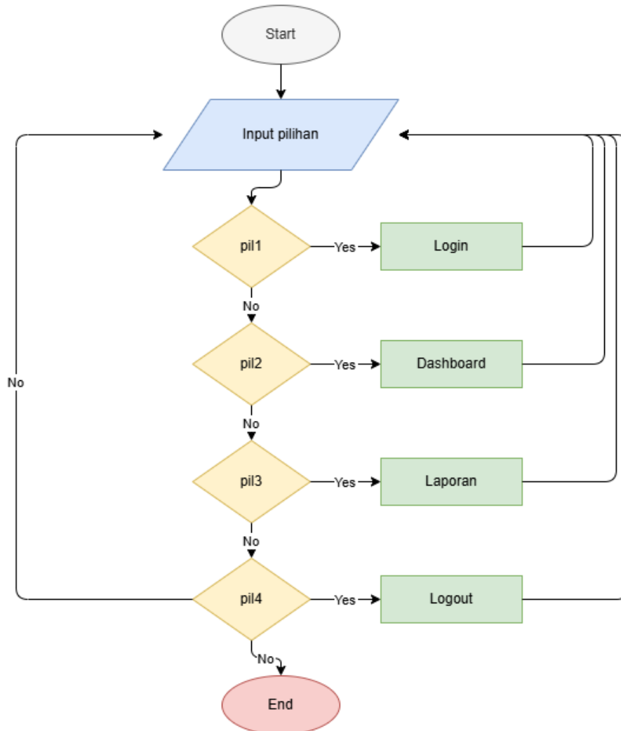
Gambar 4.50 flowchart Menu Pimpinan Sumber : Hasil Rancangan
