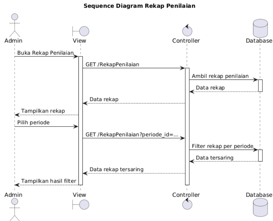
Gambar 4.27 Sequence Diagram Rekap Penilaian Sumber : Hasil Rancangan
