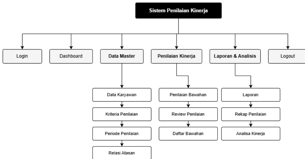
Gambar 4.34 Rancangan Struktur Menu Sumber : Hasil Rancangan
