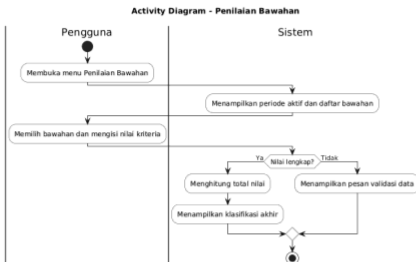
Gambar 4.14 Activity Diagram Penilaian Bawahan Sumber : Hasil Rancangan
