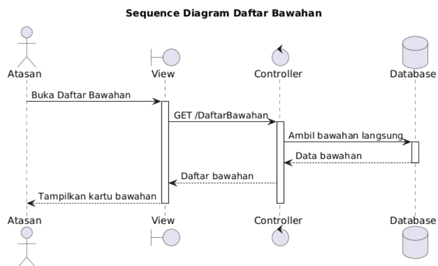
Gambar 4.31 Sequence Diagram Daftar Bawahan
