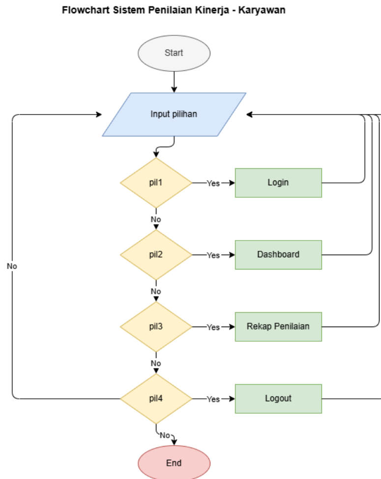
Gambar 4.49 flowchart Menu Karyawan Sumber : Hasil Rancangan
