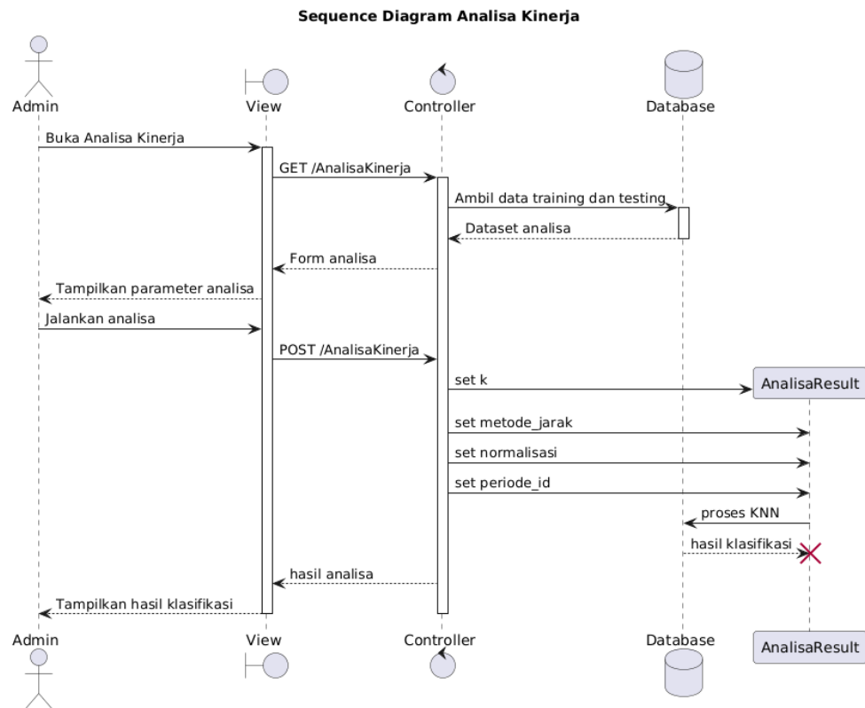
Gambar 4.28 Sequence Diagram Analisa Kinerja Sumber : Hasil Rancangan
